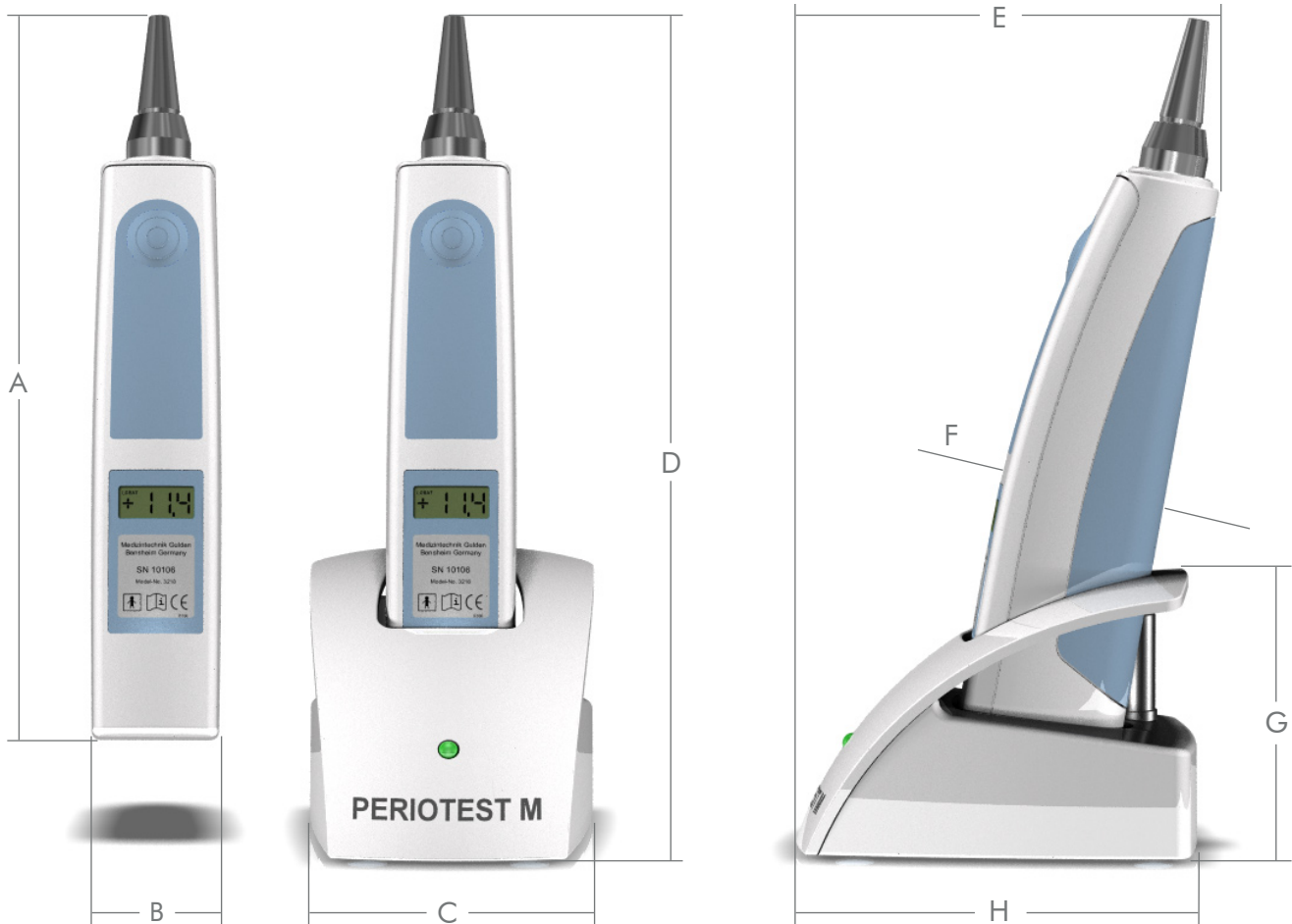
Periotest M, Typ 3218, Artikel-Nr. 8917140
